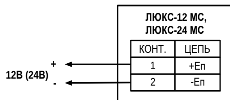
Рис.1. Схема подключения.
