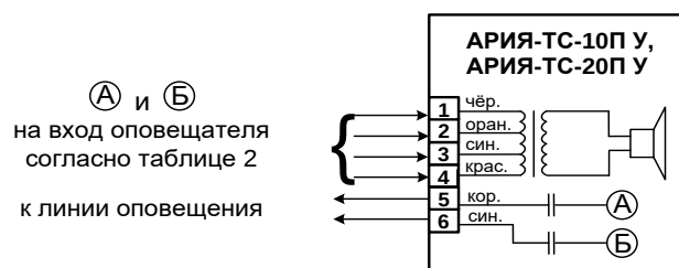
Рис. 1. Схема подключения
