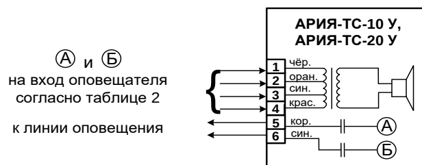
Рис. 1. Схема подключения
